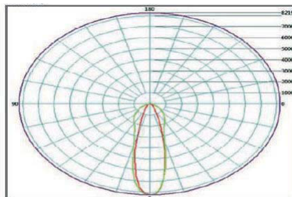
Luminous Flux OM Optic 3930lm
