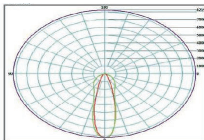
Luminous Flux OM Optic 3930lm
